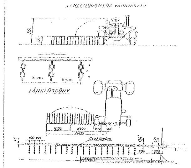
Láncfüggönyös vadriasztó
