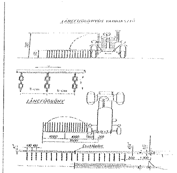
Láncfüggönyös vadriasztó
