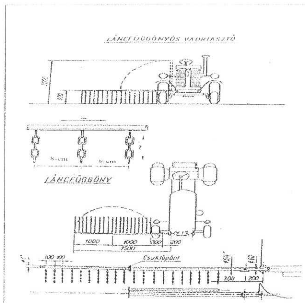
Láncfüggönyös vadriasztó
