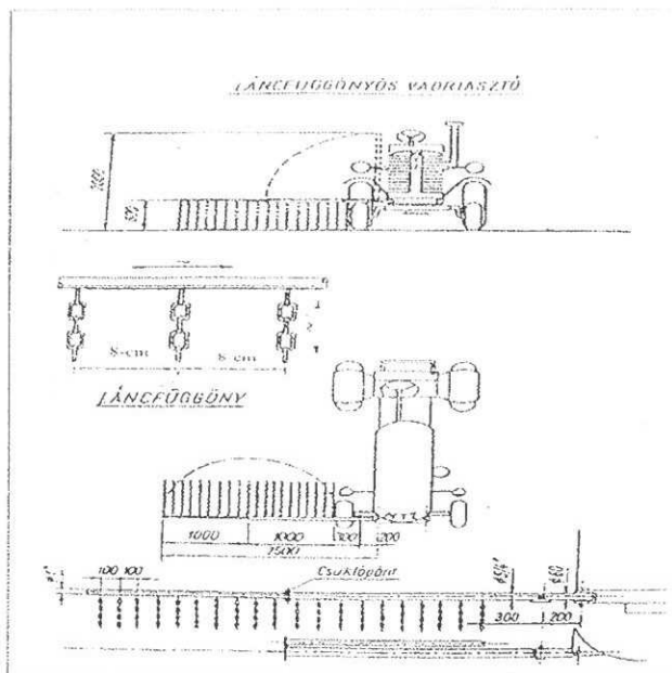
Láncfüggönyös vadriasztó
