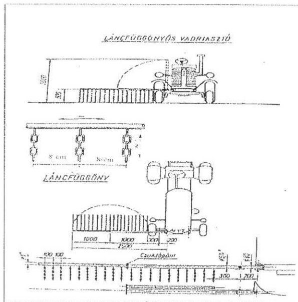
Láncfüggönyös vadriasztó
