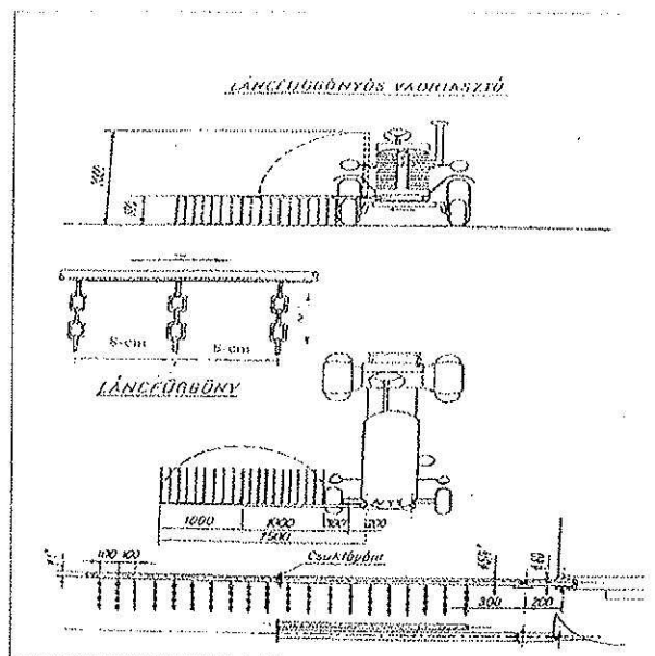
Láncfüggönyös vadriasztó
