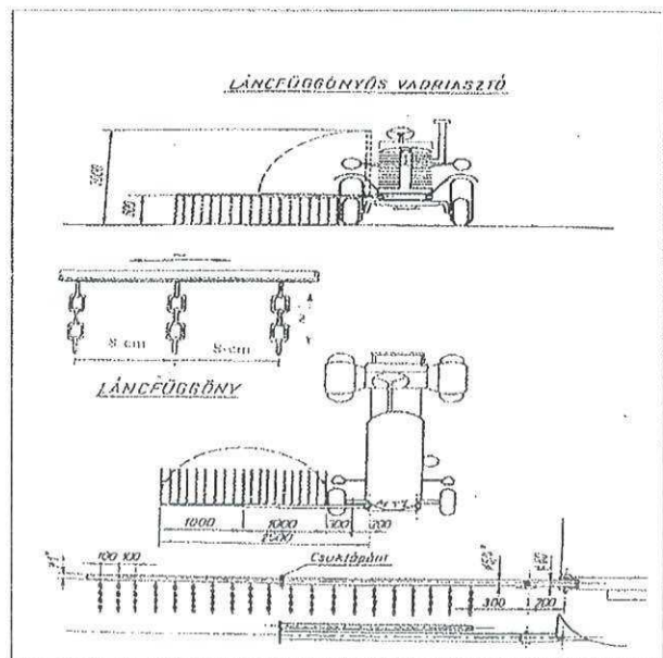
Láncfüggönyös vadriasztó
