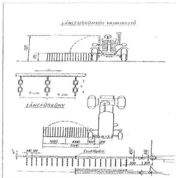
Láncfüggönyös vadriasztó
