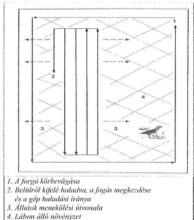
Kiszorító kaszálás
