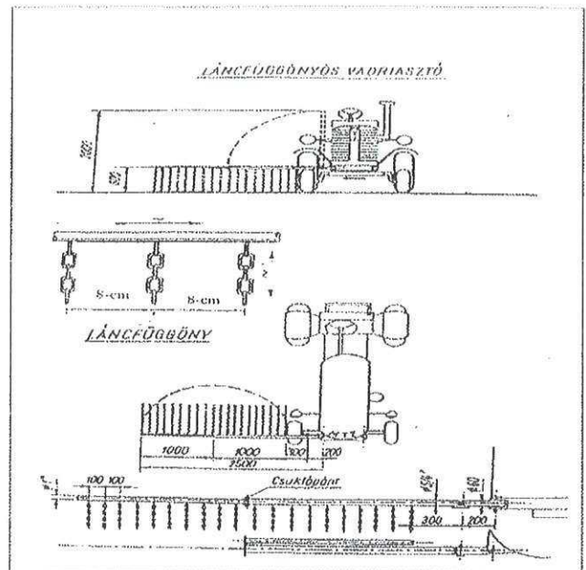
Láncfüggönyös vadriasztó
