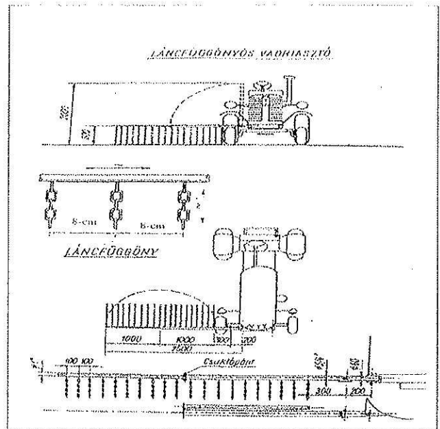
Láncfüggönyös vadriasztó
