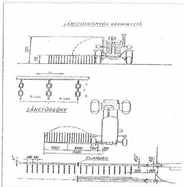
Láncfüggönyös vadriasztó
