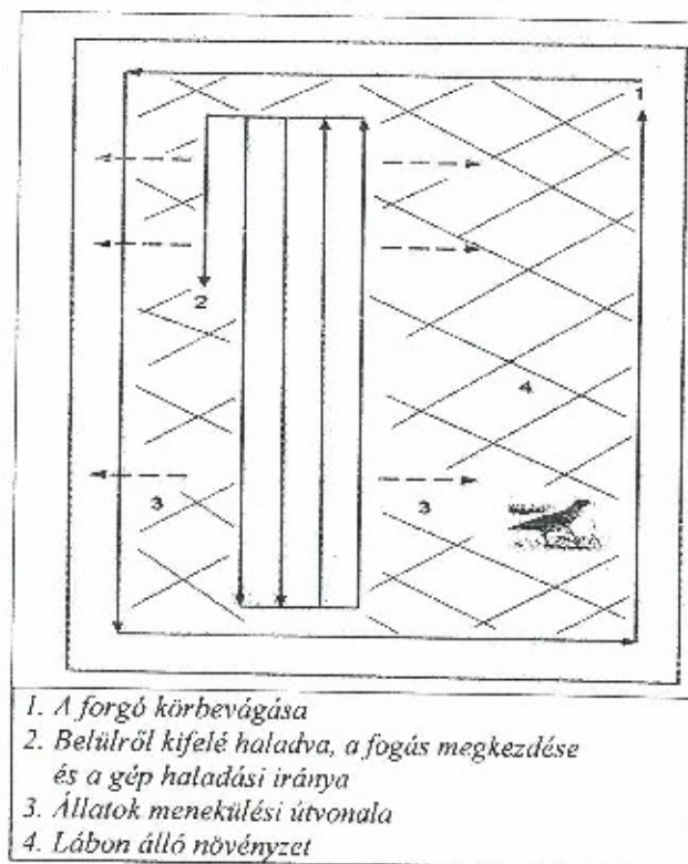
Kiszorító kaszálás
