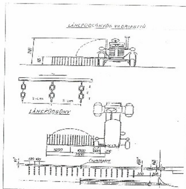
Láncfüggönyös vadriasztó
