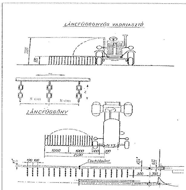
Láncfüggönyös vadriasztó
