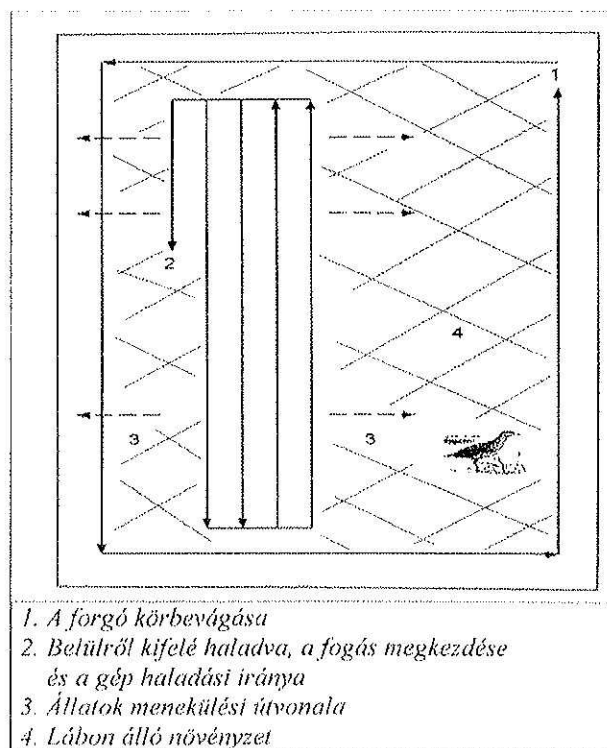
Kiszorító kaszálás
