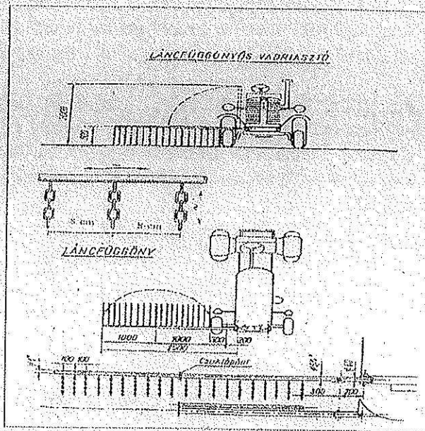
Láncfüggönyös vadriasztó
