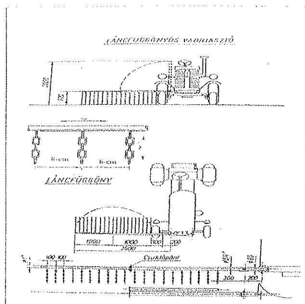
Láncfüggönyös vadriasztó
