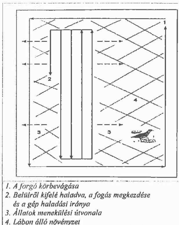
Kiszorító kaszálás
