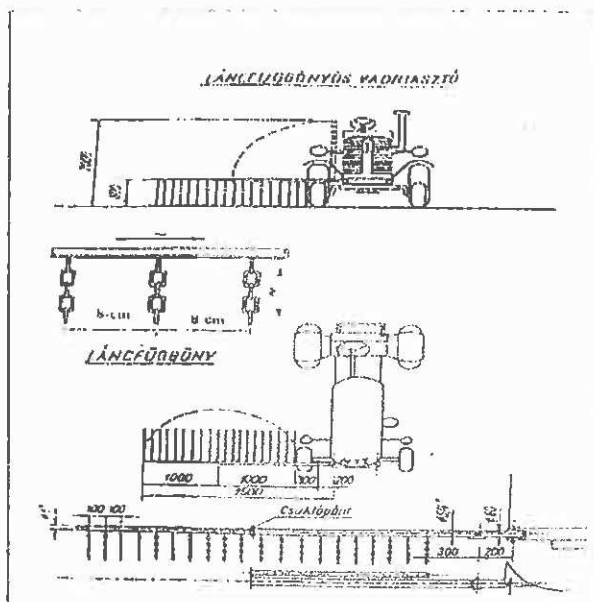
Láncfüggőnyös vadriasztó
