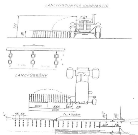
Láncfüggönyös vadriasztó
