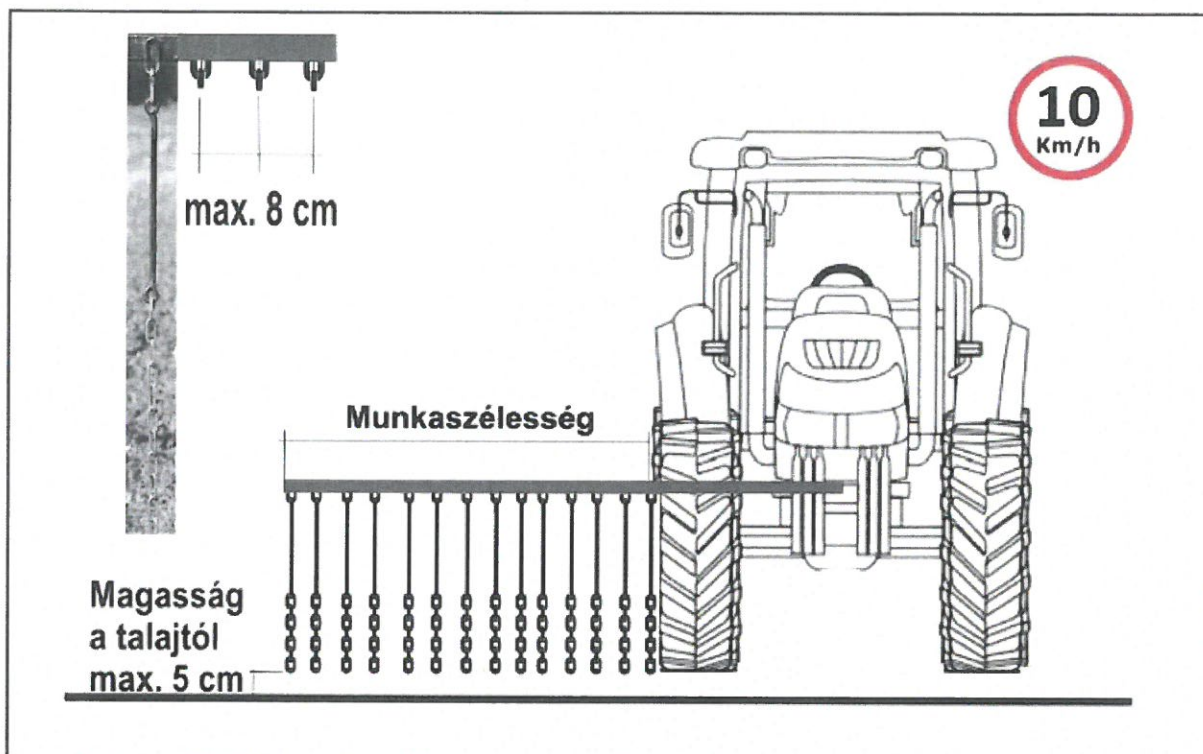
Láncfüggönyös vadriasztó
